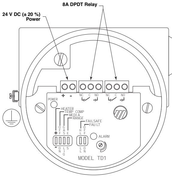
TD1 Wiring
